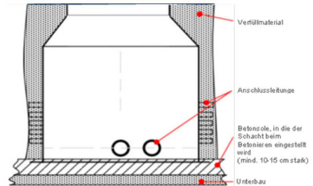
Abb. 1: Schematische, beispielhafte Darstellung der Einbausituation
