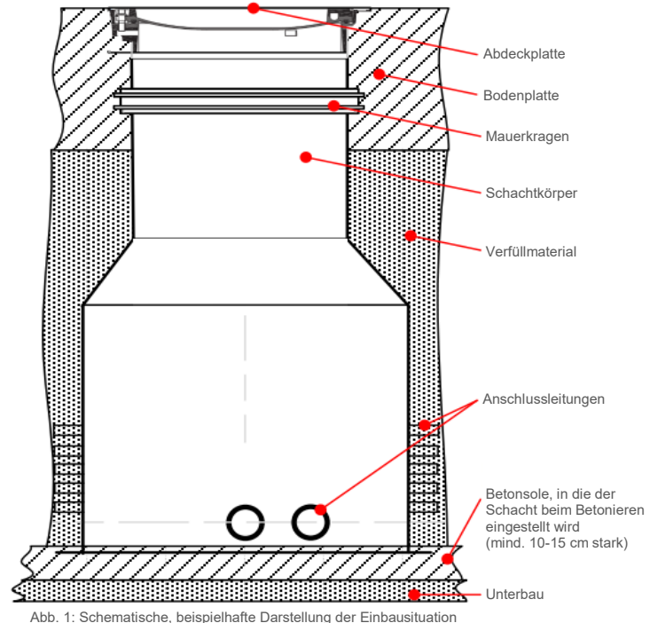
Abb. 1: Schematische, beispielhafte Darstellung der Einbausituation
